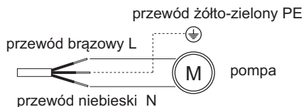
Rys. 4 Schemat podłączenia przewodu do pompy
